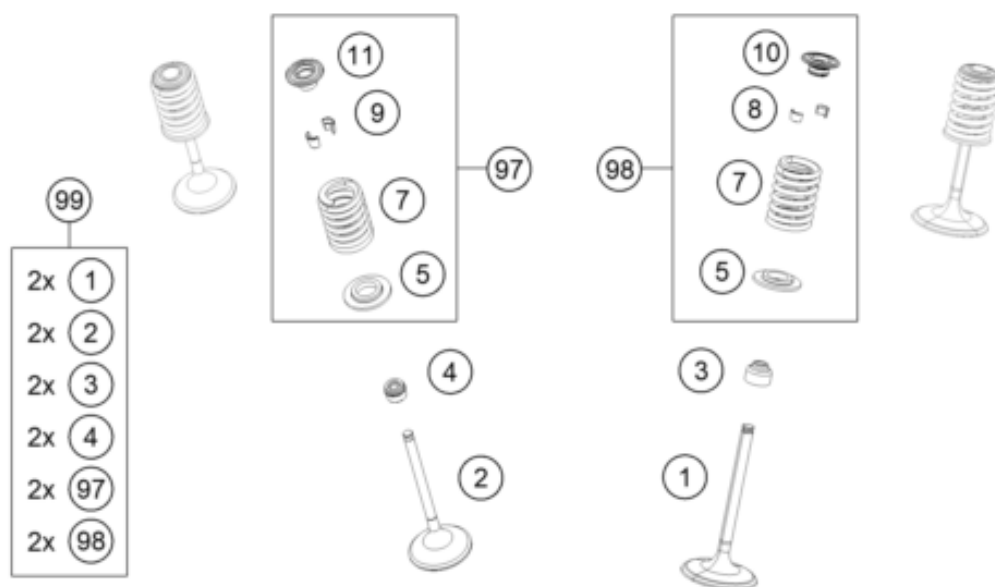
AUSLASS / EXHAUST
